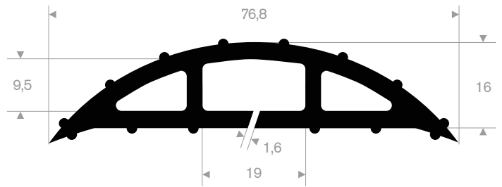
215.00.471 PVC black roll length 9 meter
