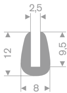
211.01.201GR TPE 70° Shore grey roll length 100 meter
