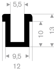
211.01.028 EPDM 70° Shore black roll length 50 meter
