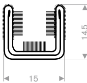
219.01.021 EPDM + textile roll length 30 meter
