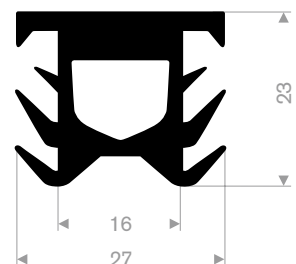
216.05.277 EPDM 70° Shore black roll length 25 meter
