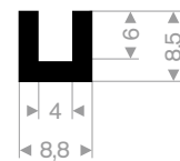
211.00.421 EPDM 70° Shore black roll length 100 meter
