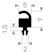
216.03.641 EPDM 70° Shore black roll length 100 meter
