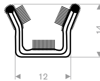
219.01.022 EPDM + textile roll length 30 meter
