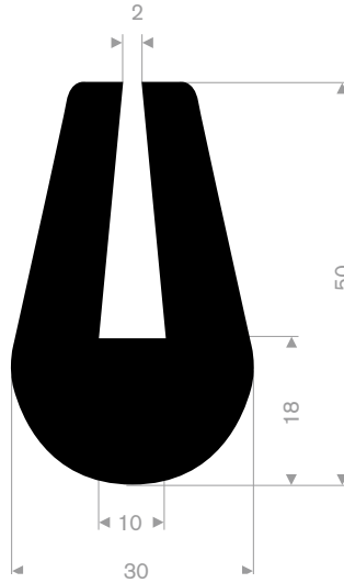
211.05.381 EPDM 70° Shore black roll length 20 meter
