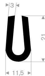
211.00.224 EPDM 70° Shore black roll length 50 meter
