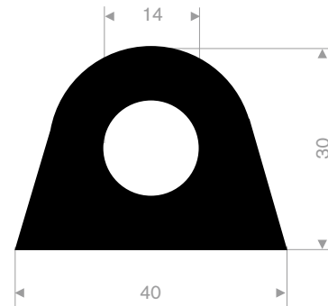
215.14.031 EPDM 65° Shore black roll length 20 meter
