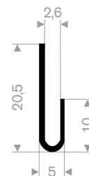
211.00.123 EPDM 70° Shore black roll length 50 meter
