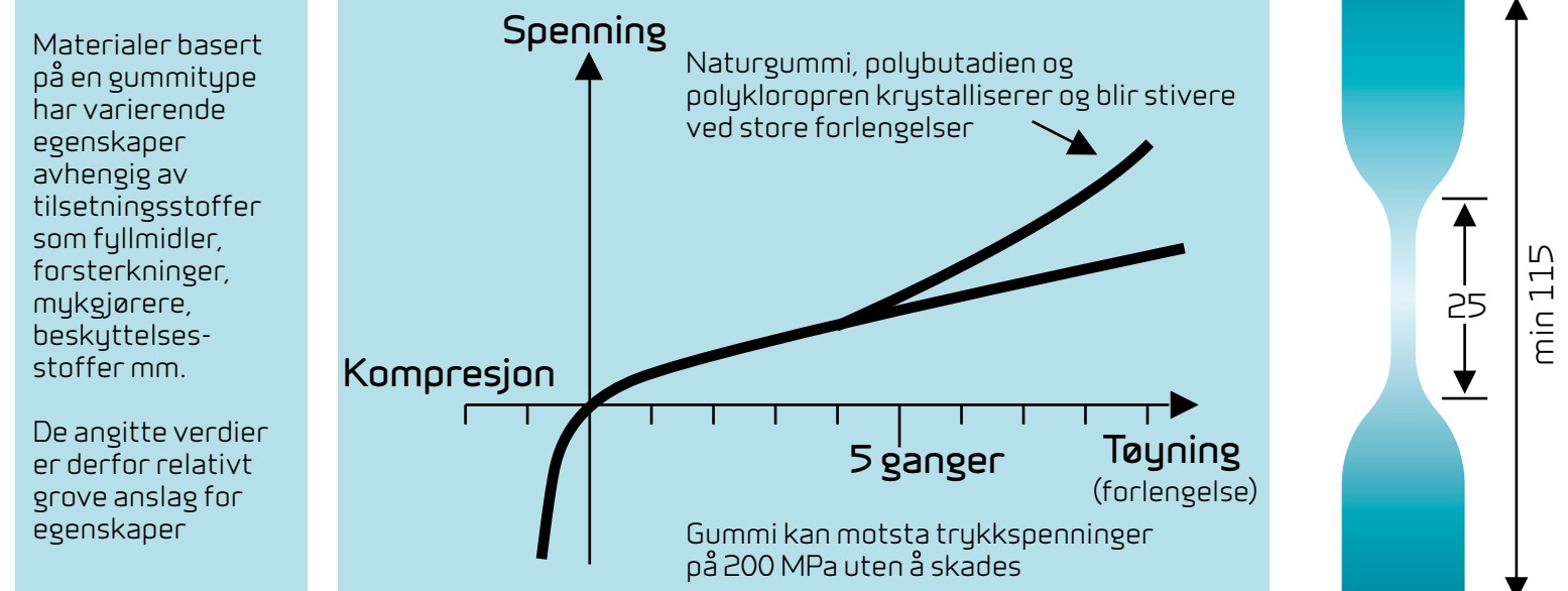
PRØVESTYKKE FOR GUMMI Tykkelse 2mm. Stivhet er vanligvis gjengitt med strekkstyrke i tøyning på 100%, 200%, 300% osv
