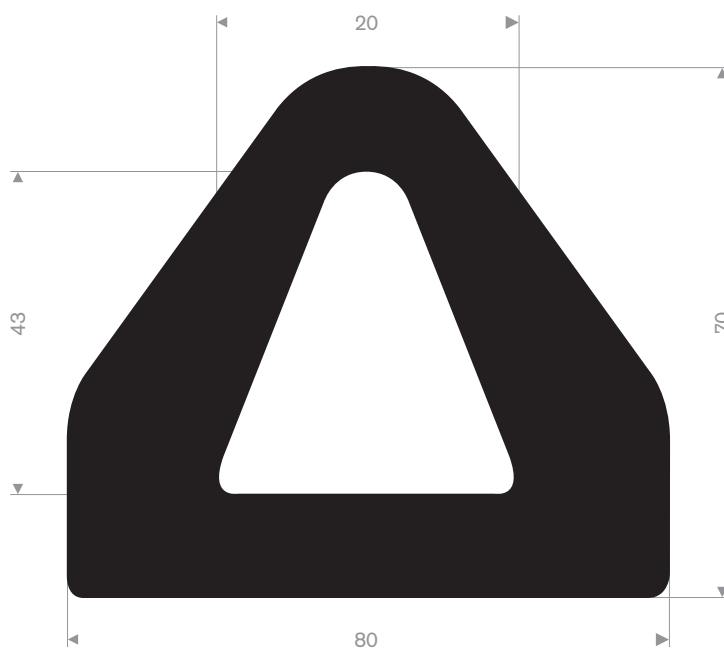
215.28.070 EPDM 70° Shore sort rull lengde 10 meter
