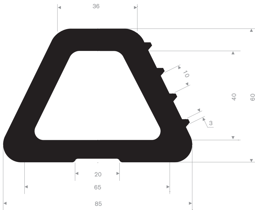
215.08.560 EPDM 70° Shore sort rull lengde 6 meter
