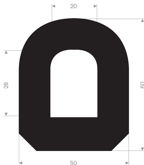
215.15.060 EPDM 70° Shore sort rull lengde 10 meter
