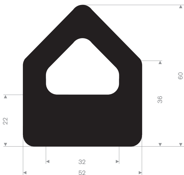
215.65.260 CR 50° Shore sort rull lengde 5 meter
