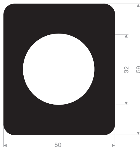
215.06.052 EPDM 70° Shore sort rull lengde 10 meter
